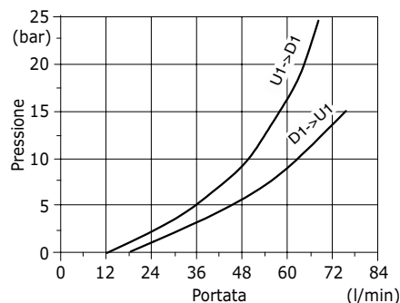
Diagramma perdite di carico VOSL/SC 12 D1->U1 e U1->D1
